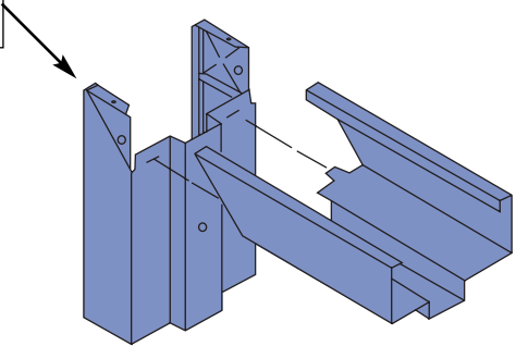
Drywall Frame Mitered
